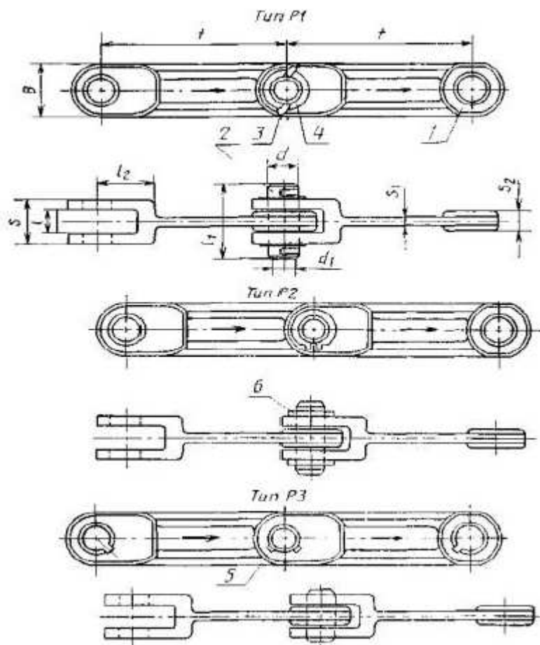
1 - звено; 2 - палец; 3 - шплинт; 4 - шайба; 5 - штифт-шпонка; 6 - сжимная стопорная шайба
